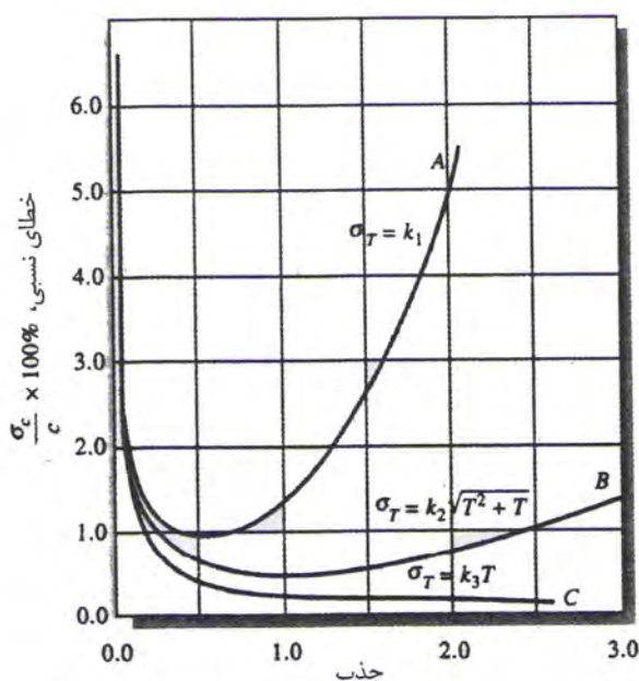
شکل ۱۰-۲۶ منحنی های خطا برای طبقه بندی های مختلف عدم قطعیت های دستگاهی.
